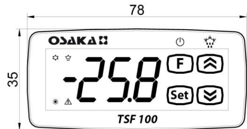
Modelo TSF 100
